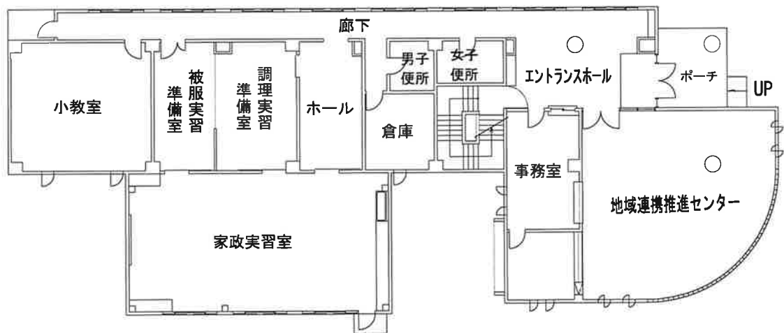
1階平面図
