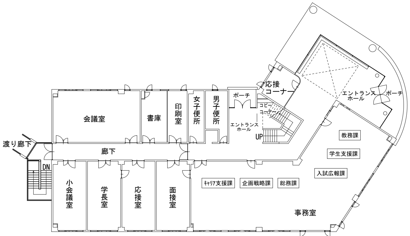
1階平面図
