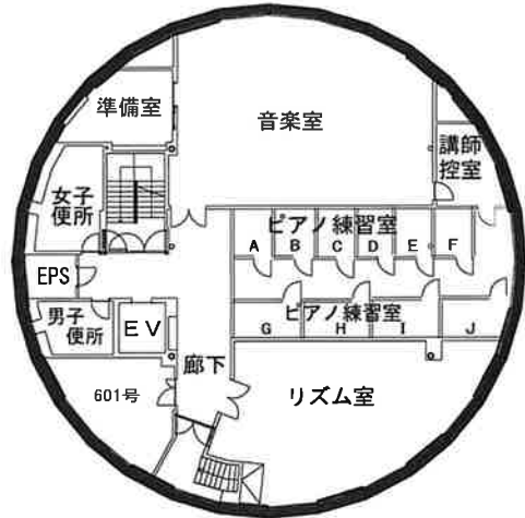
6階平面図
