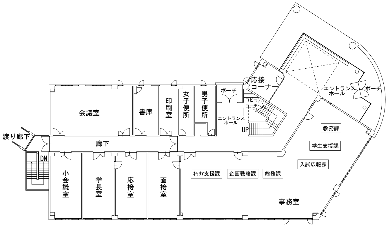
1階平面図
