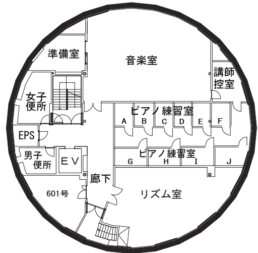
6階平面図
