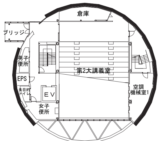
2階平面図
