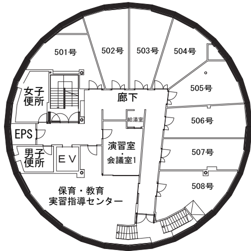
5階平面図
