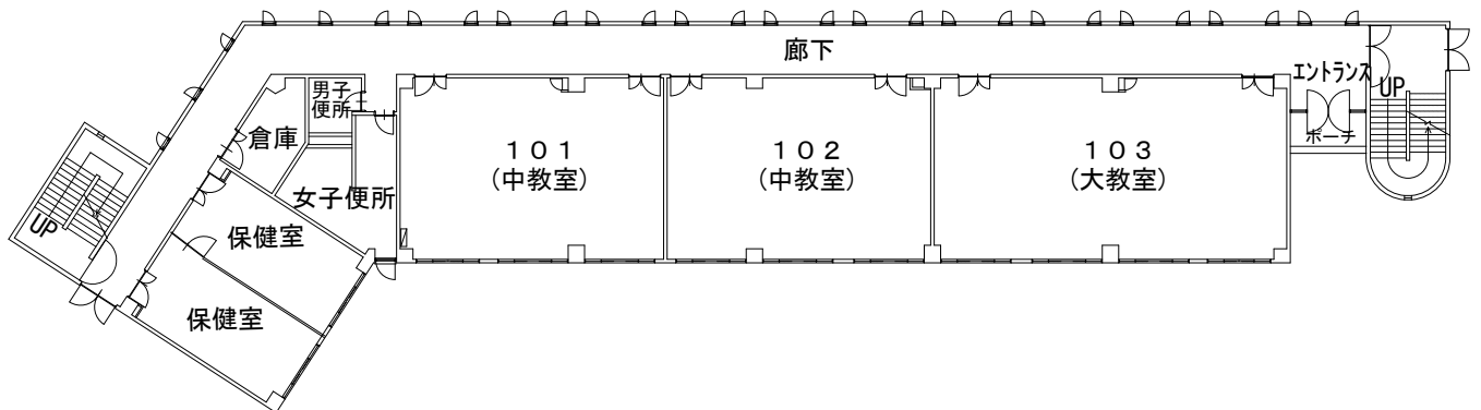
1階平面図
