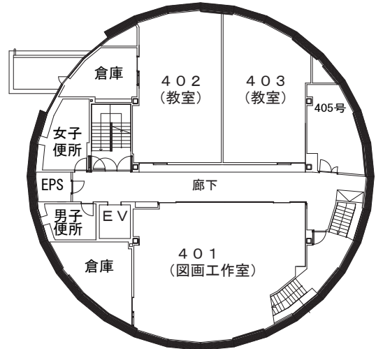
4階平面図
