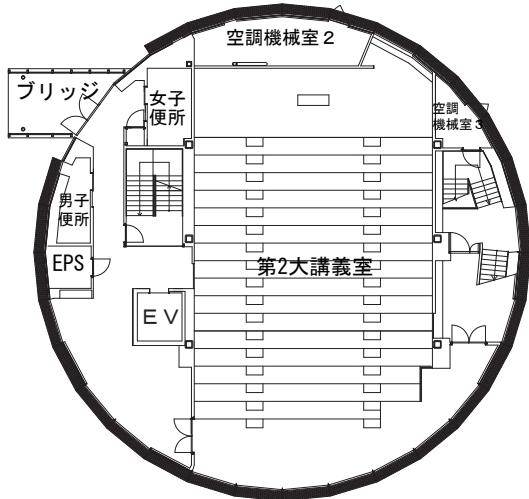
3階平面図
